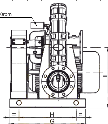
Wersja z połączeniem pasowym
